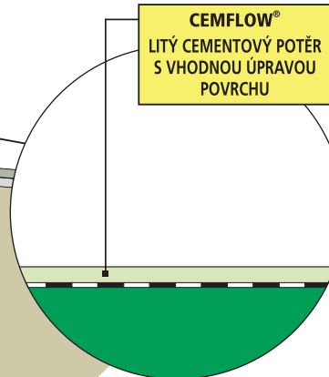
Detail podlahového souvrství garáž, sklep
