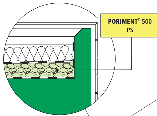
Detail ploché střechy
