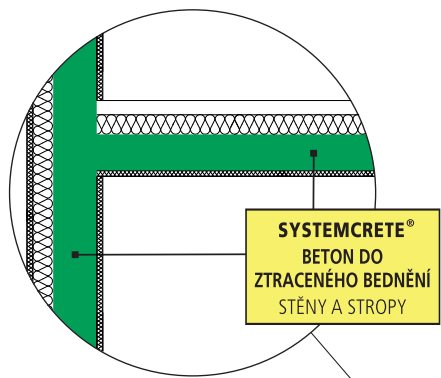
Detail svislé a stropní konstrukce
