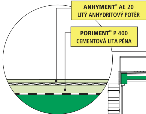
Detail podlahového souvrství obytná část
