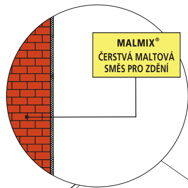
Detail zděné svislé konstrukce
